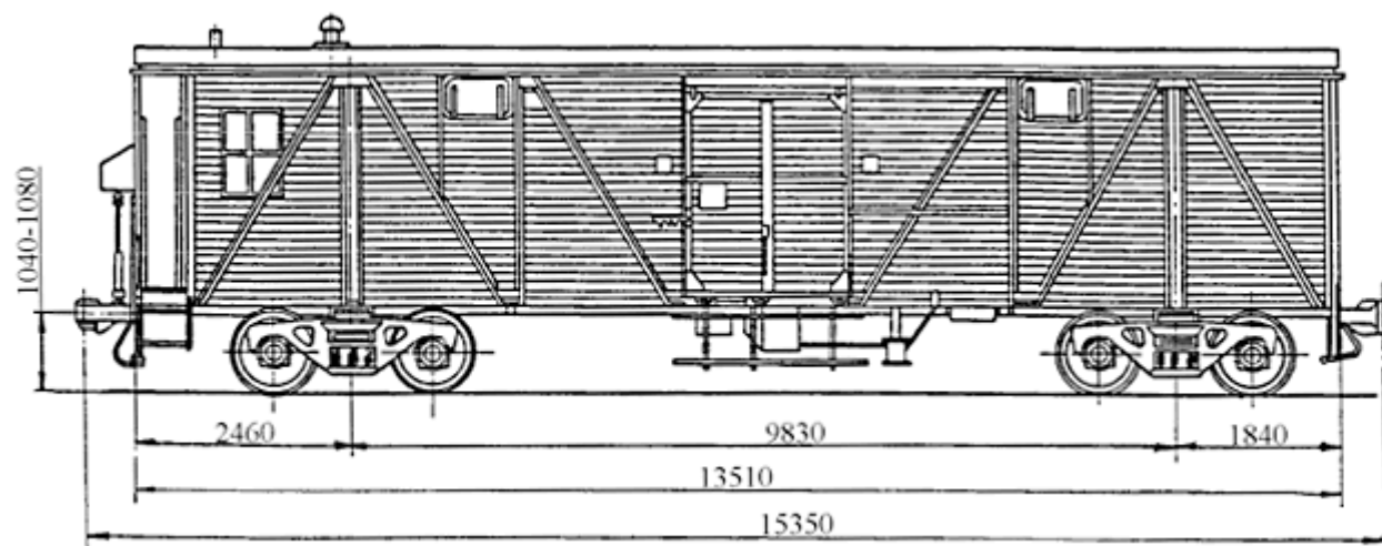
Сборно-раздаточный вагон
